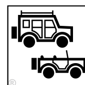
SAMOCHOODY TERENOWE
